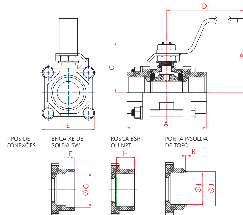
VÁLVULA DE ESFERA TRIPARTIDA PASSAGEM REDUZIDA (PR)
